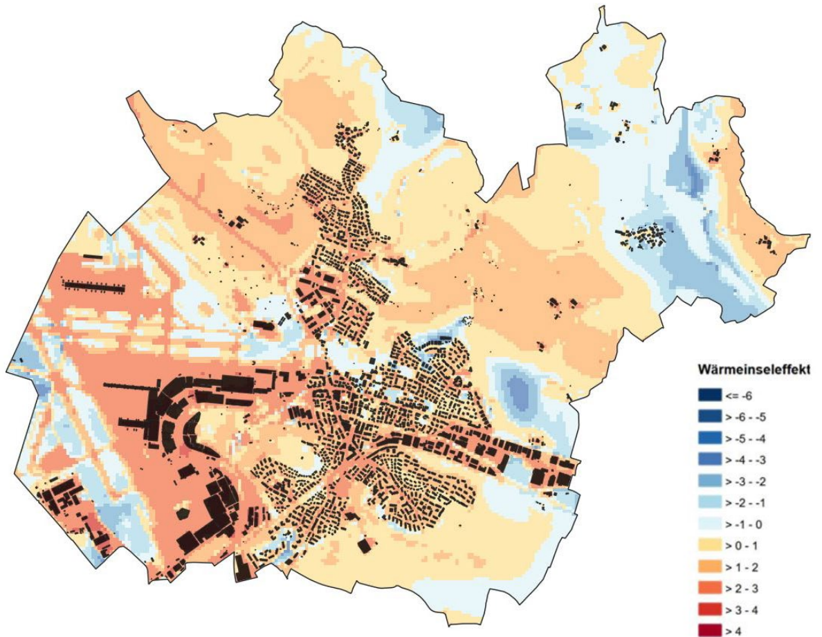
Abb. 6.1 Klimaanalysekarte Nacht - Wärmeinseleffekt.
